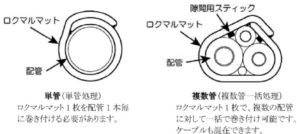
図-1 ロクマルマットの巻付け条件
