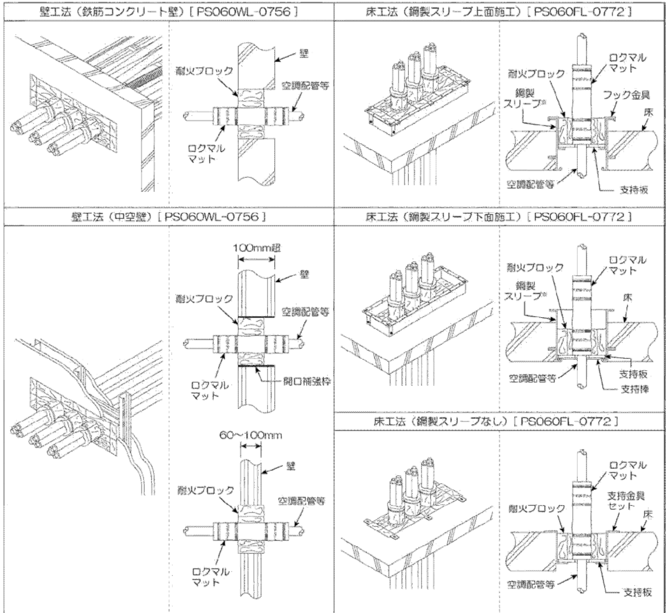
図-2 施工例
