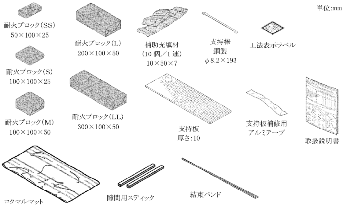
図-3 キット品の構成材料の一覧
