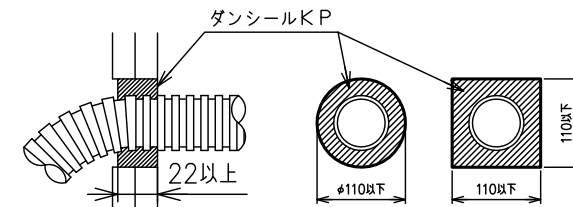
開口B詳細図
