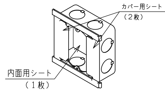
ボックス部詳細
