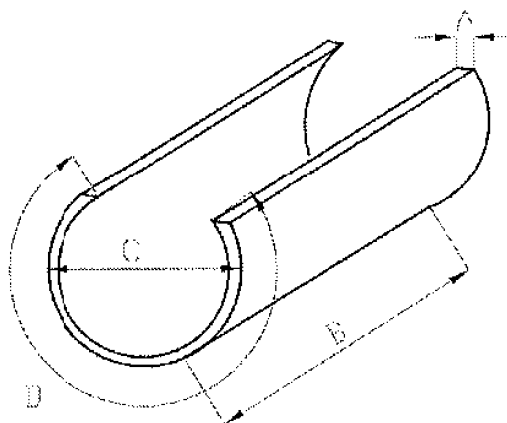
図-1 熱膨張材
