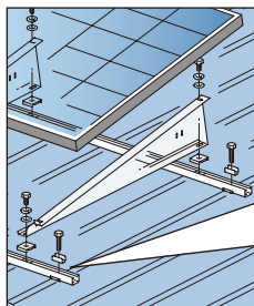
架台取付図
