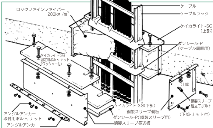
タフロック ニジカン ウエカラ仕様書 (単位mm 高さは全サイズ 200mm)
