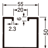
AD-5断面図
