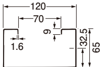
DP-12断面図
